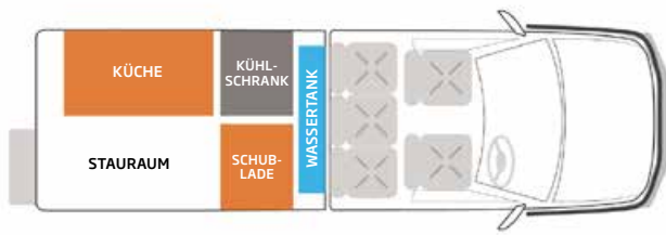
Anordnung des Fahrzeugaufbaus
