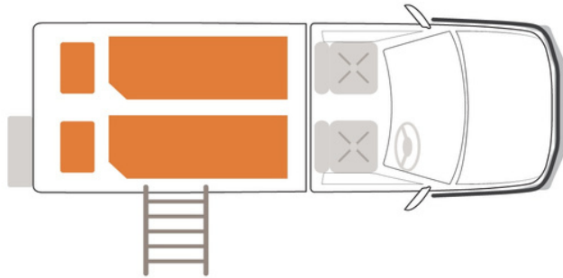
Anordnung des Fahrzeugaufbaus
